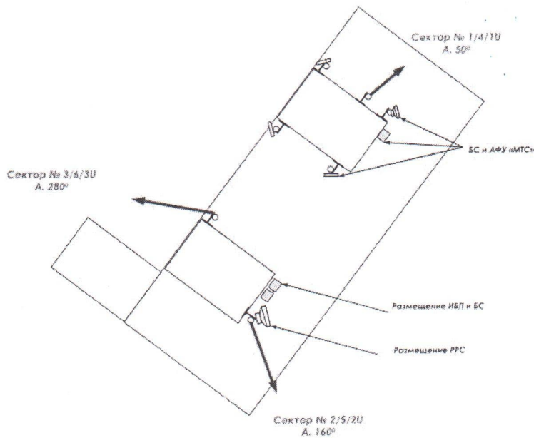
Схема размещения АФУ
